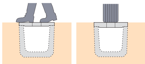
1種 輪荷重を受けない場所 2種 輪荷重 T-8 (32KN以下)
