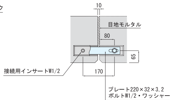
接続金具部詳細図
