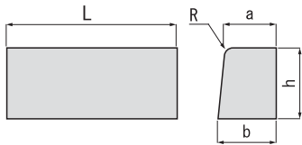
JIS A5371 歩車道境界ブロック
