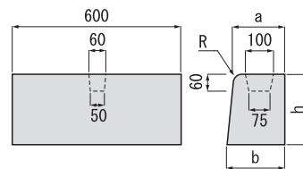
セパレーター
