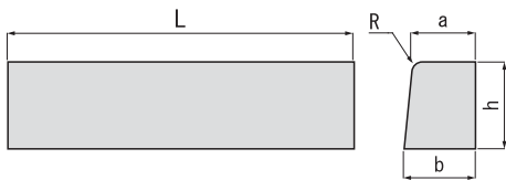
歩車道境界ブロック
