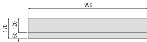
■ PCC-A 橋梁用ネジ込み式 参考重量：64kg
