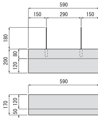
■ PCC-A ネジ込み式 参考重量：38kg
