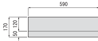
■ PCC-A 参考重量：38kg
