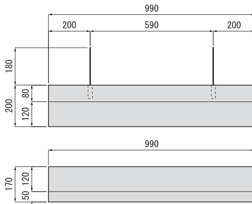
■ PCC-A 橋梁用ネジ込み式 参考重量：64kg
