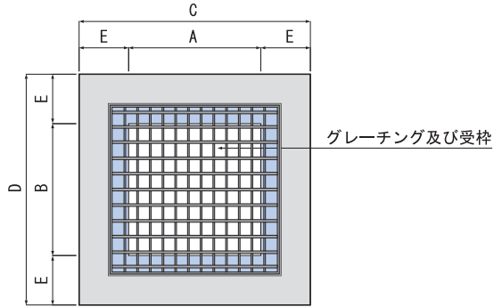
■角柵（グレーチング付）
