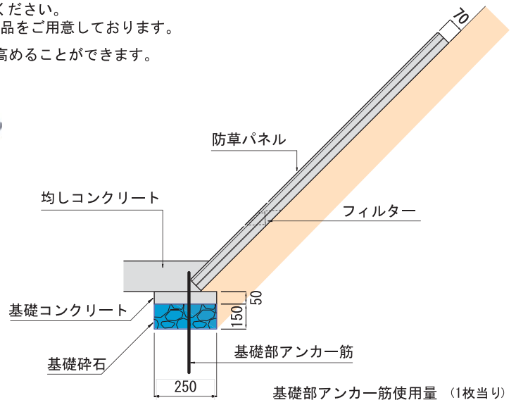
基礎部アンカー筋使用量 (1枚当り)
