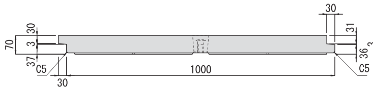
■防草パネル (法尻用) 参考重量260kg
